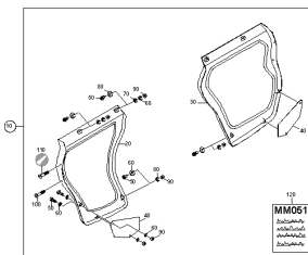
ETB-0000004976, Osłona przeciwbłotna
