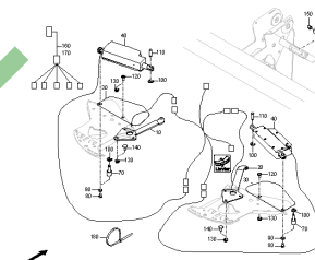
ETB-0000004179, Pakiet elektroniki Easy 2
