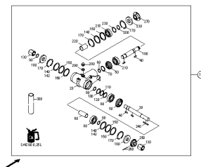
ETB-0000004078, Przekładnia wejściowa
