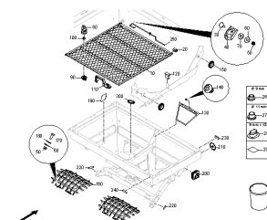
ETB-0000004061, Rama i zbiornik - sito / krata ochronna
