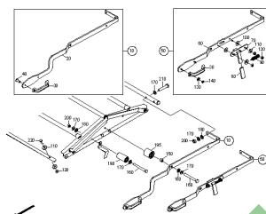
ETB-0000004205, Składana plandeka, dźwignia ręczna
