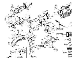
ETB-0000004920, Ekran rozszewu granicznego - limiter le. / pr.
