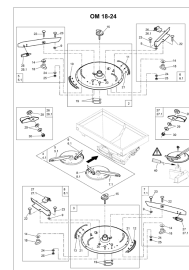
ETB-000921, Tarcza rozszewająca OM 18-24
