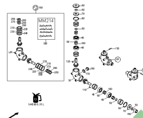
ETB-0000004084, Przekładnia kątowa le./pr.
