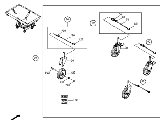
ETB-0000004798, Kółka transportowe hamowane
