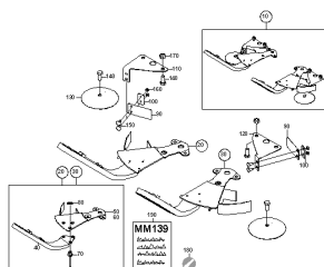
ETB-0000004939, Zestaw do rozszewu na zboczach
