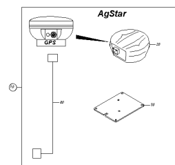
ETB-0000004983, Pakiet odbiornikowy GPS AG-Star
