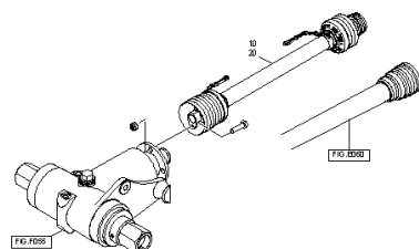
ETB-0000004967, Wałek przekąźnikowy
