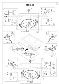
ETB-000920, Tarcza rozszewająca OM 10-16
