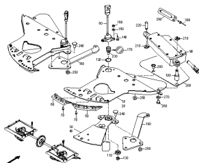
ETB-0000004072, Dno z otworami Easy 2
