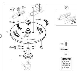
ETB-0000004915, Tarcza do rozszewu granicznego TS 10-14 lewa
