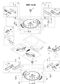
ETB-000923, Tarcza rozszewająca OMT 10-28
