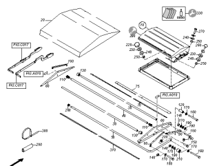
ETB-0000004198, Składana plandeka
