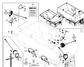
ETB-0000009399, Zestaw oświetlenia roboczego
