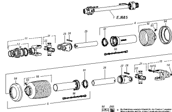
ETB-0000005669, Wałek przegubowo-teleskopowy EJ685 - SD05, 810 mm, z widelcem Russia
