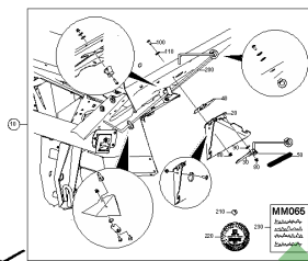
ETB-0000004942, Urządzenie do ustawiania odpowiedniej dawki rozsiewu
