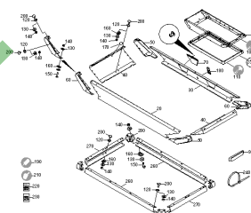
ETB-0000004155, Nadstawka S 502 / L 1002
