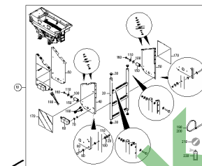
ETB-0000004809, Oświetlenie obrysowe przednie / drabina
