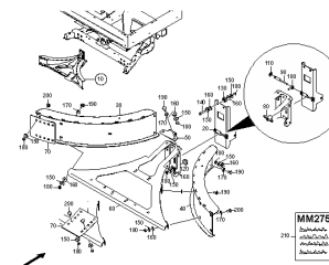
ETB-0000004973, Ekran rozszewu krawędziowego lewy
