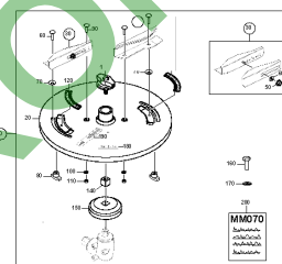
ETB-0000004916, Tarcza do rozszewu granicznego TS 15-18 lewa
