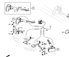
ETB-0000004992, Pakiet elektroniki EasySet
